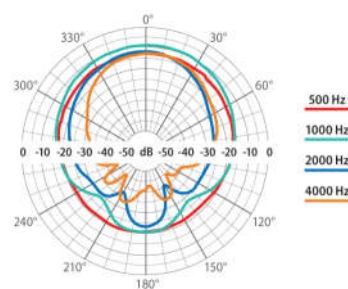
Suuntakuviön ympyräkaavio – pystysuora:
