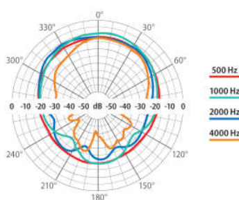
Suuntakuviön ympyräkaavio – vaaka:
