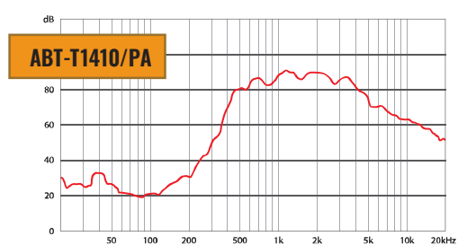
Taajuuskaista
