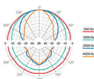
Suuntakuviön ympyräkaavio:
